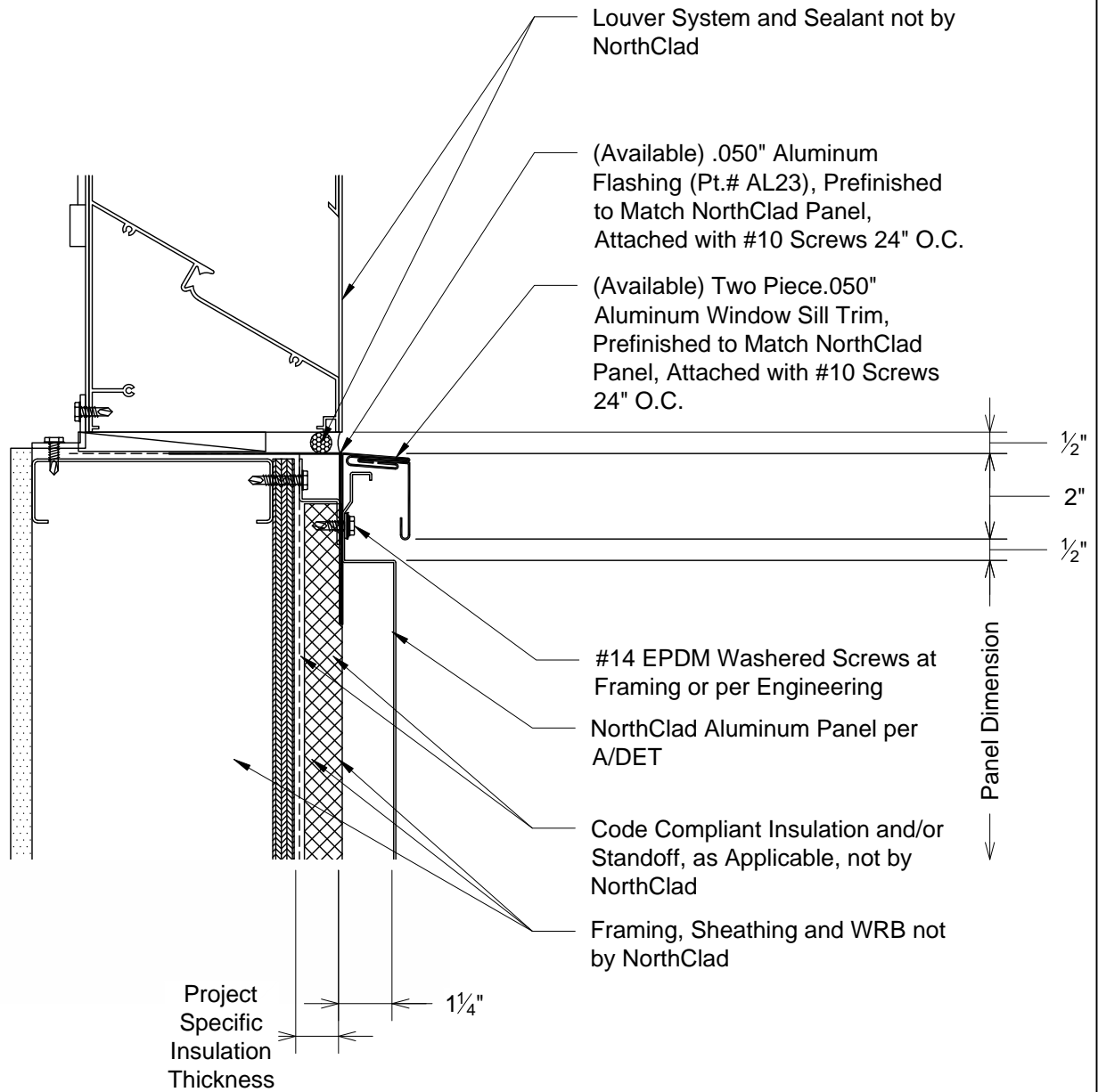
N2 Section - Louver Sill DET
