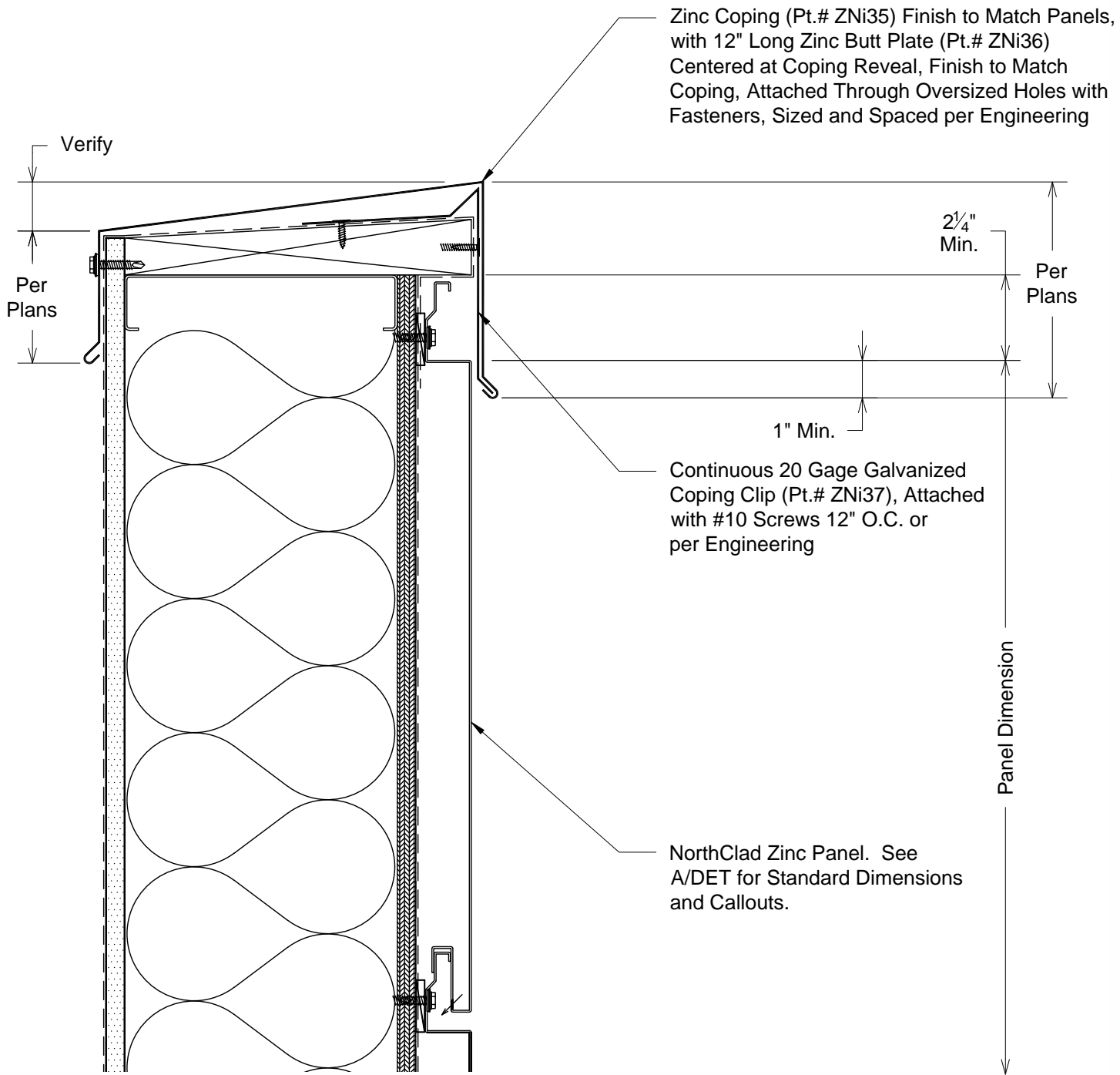
D Section - Parapet Coping DET
