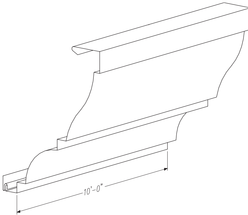
GS 650 COR CORNICE FASCIA
