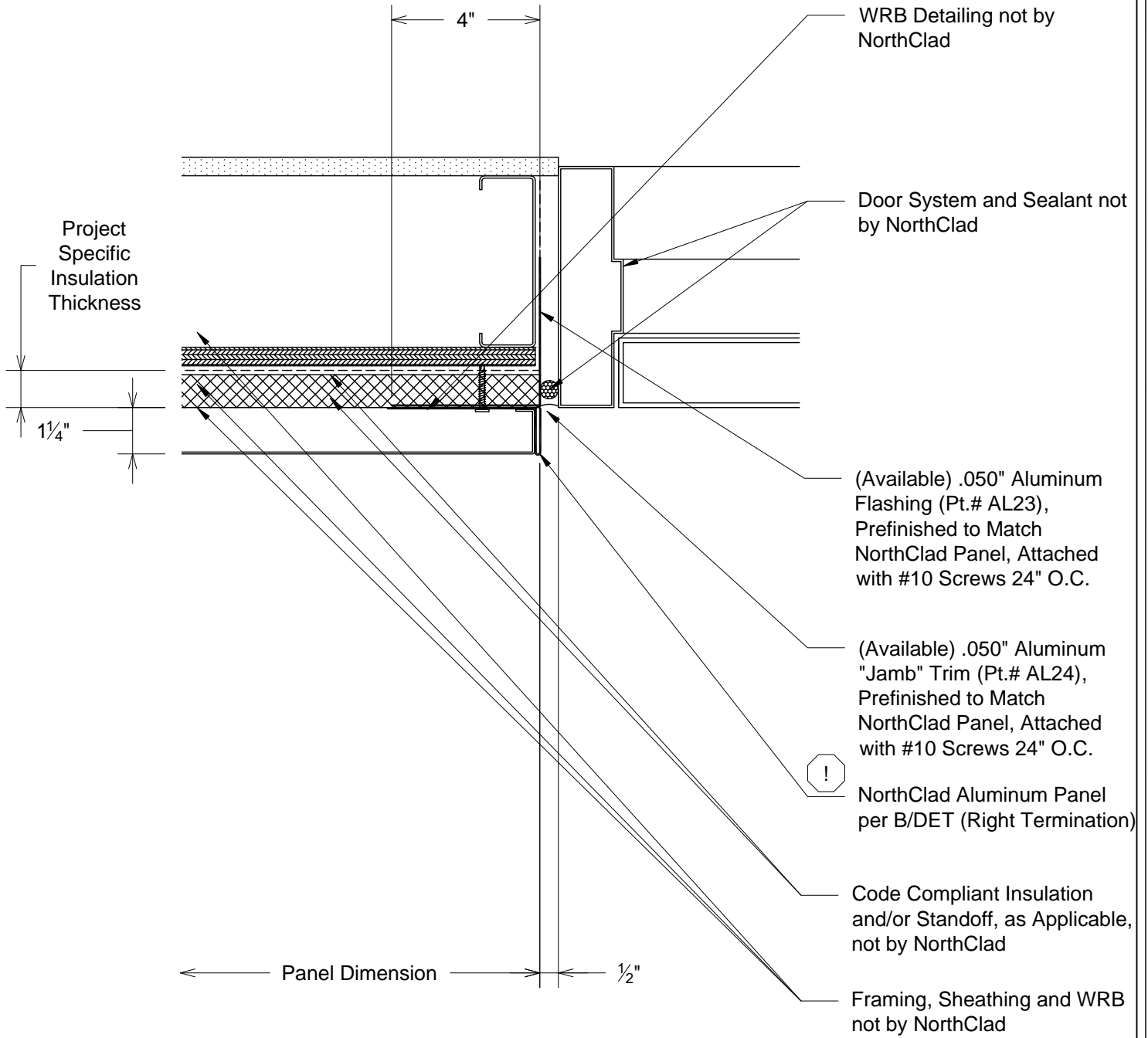
K3 DET Plan - Door at Left Jamb
