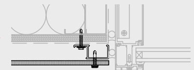
Window Jamb
