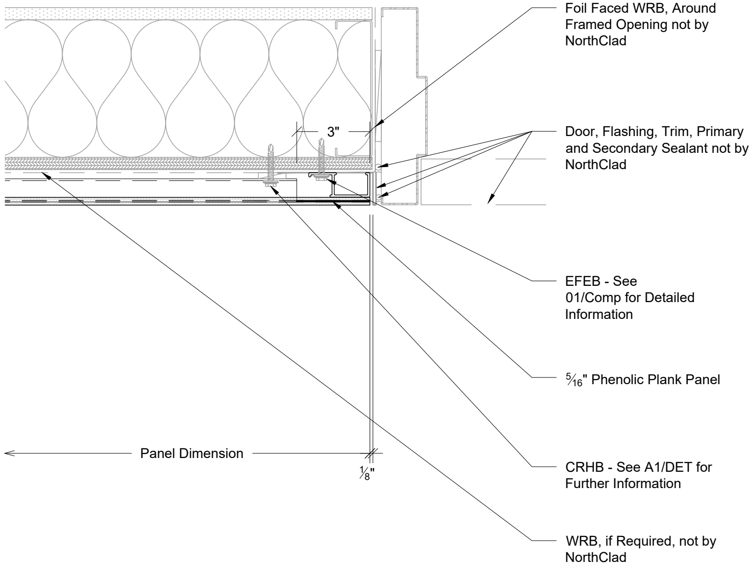
Plan - Door at Left Jamb
